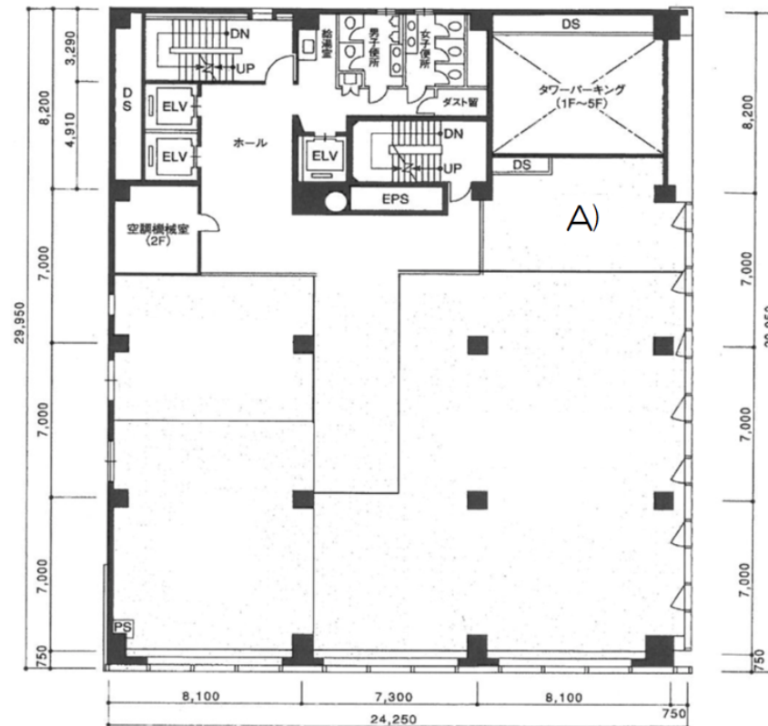
桂和大通ビル50 2階平面図 平面図…A)のスペース
