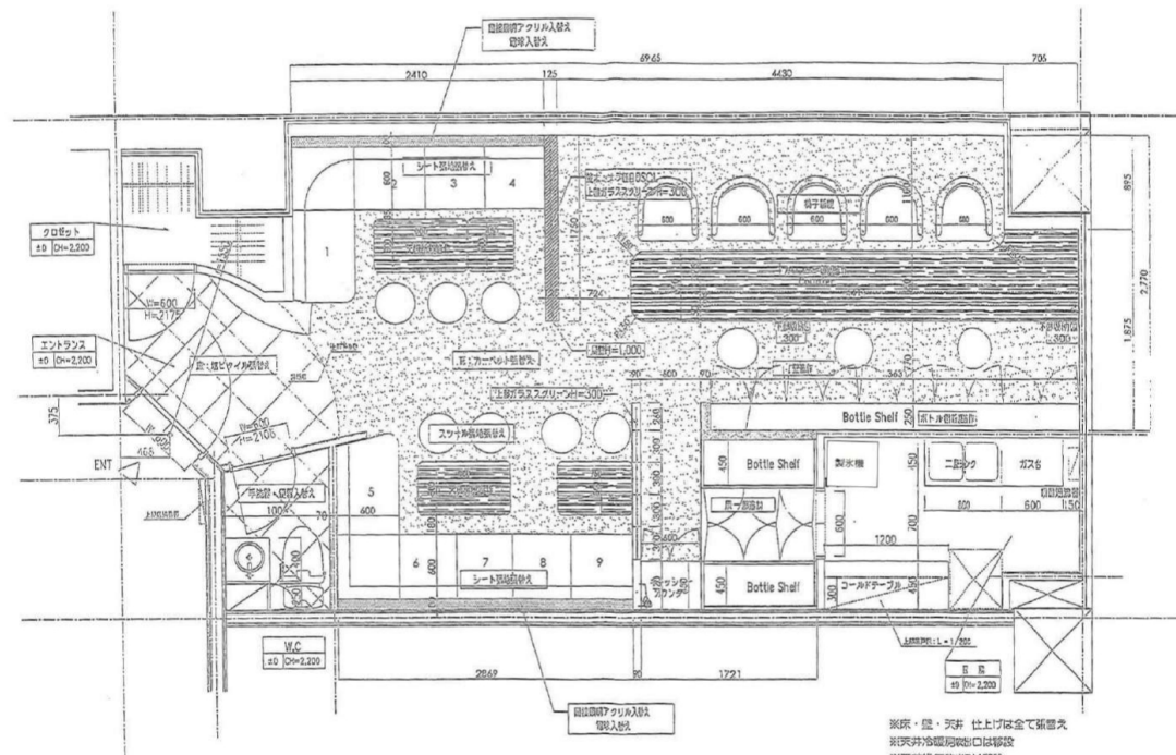
第20桂和ビル5階3号 平面図
